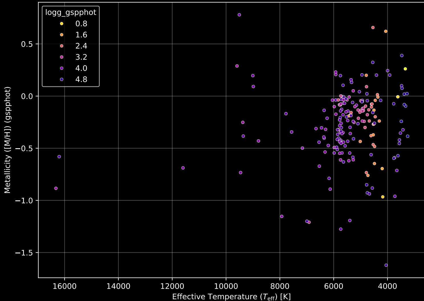
APOGEE DR17 Field: [K2_C7_020-17_btx] Stellar Population Parameters (n= 196)
